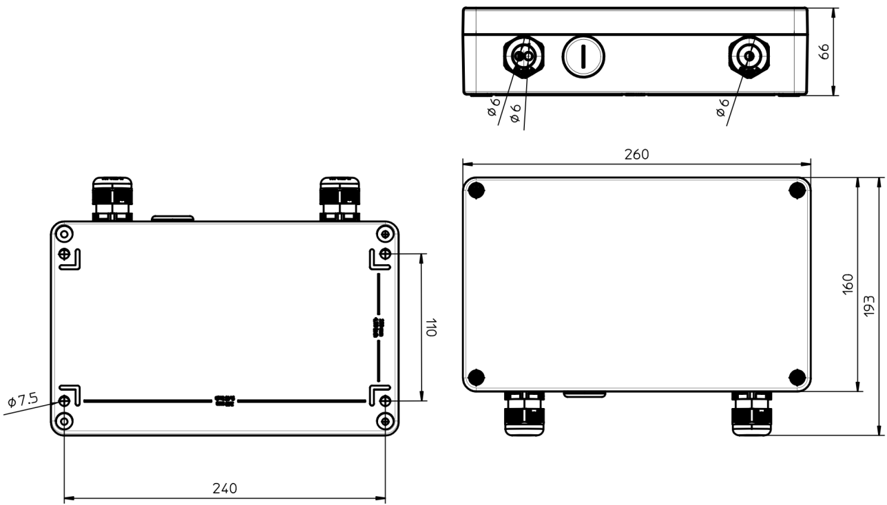
Abbildung 1: Abmessungen
