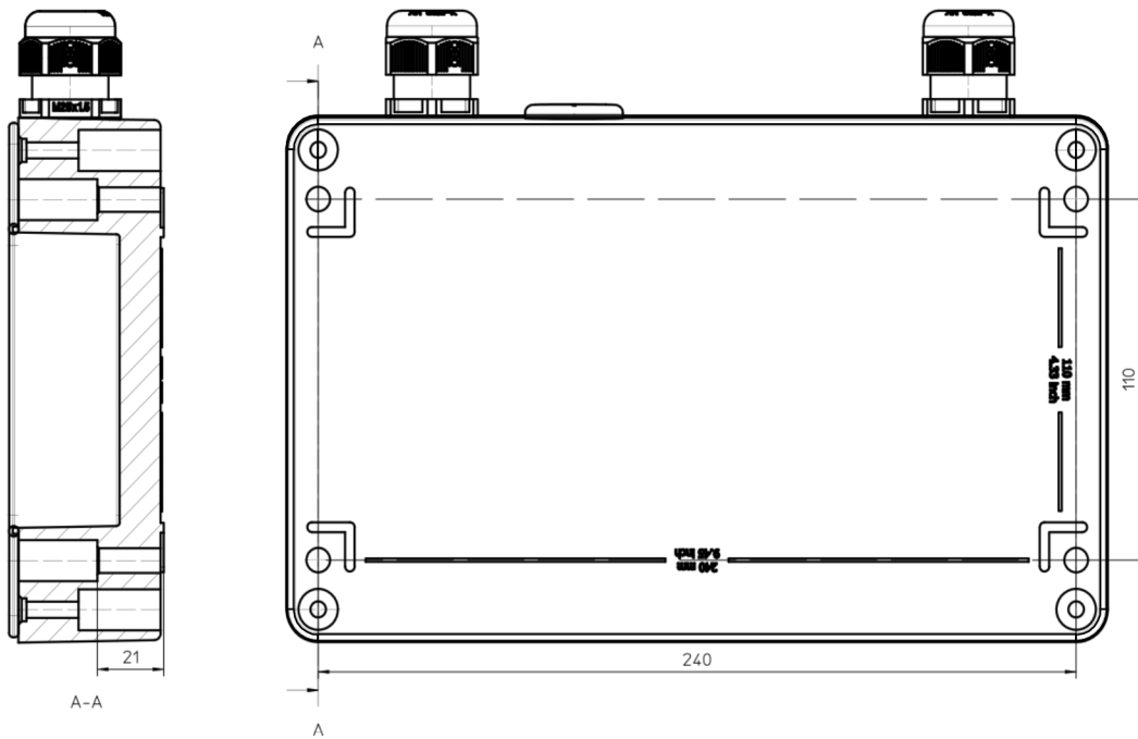
Abbildung 2: Bohrungen
