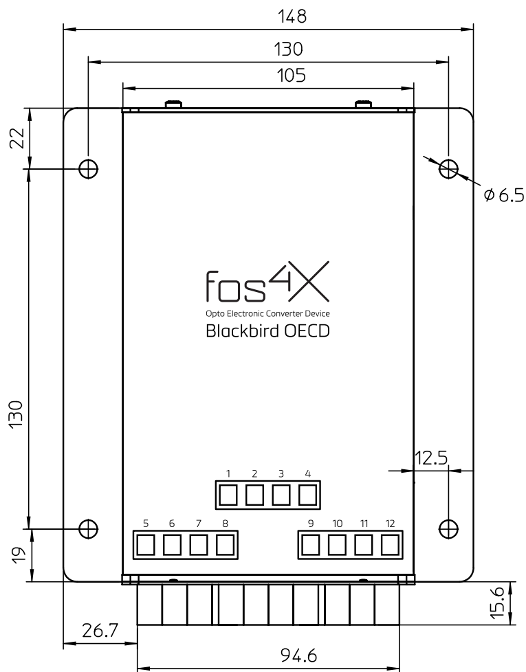
Abbildung 1: Abmessungen (Ansicht von oben)
